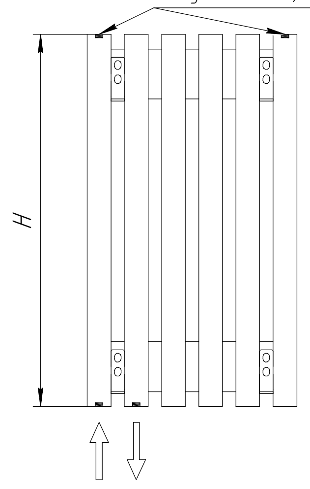
Воздухоотводчик G1/2
