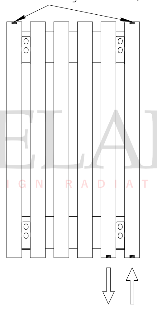
Воздухоотводчик G1/2
