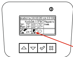
Разъем OpenTherm
