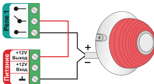
Схема подключения к релейному выходу:
