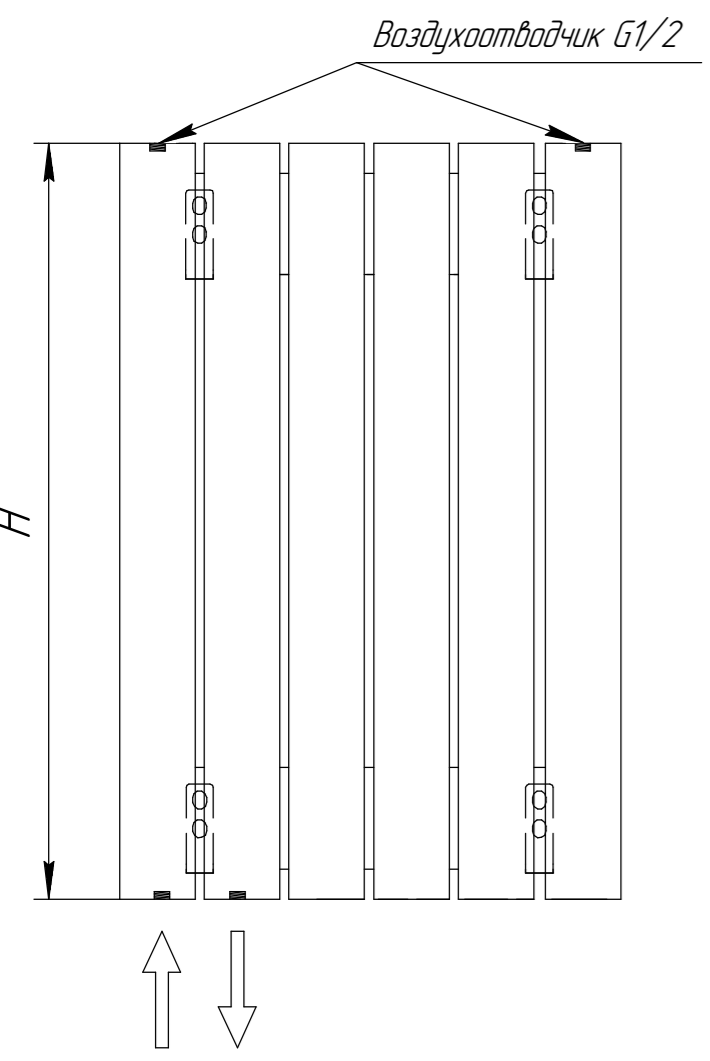
Подключение нижнее "биноклем" 150
