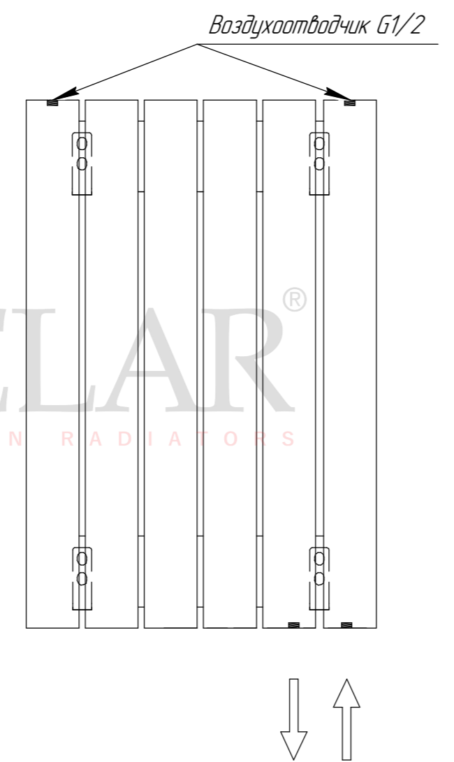
Подключение нижнее "биноклем" 150
