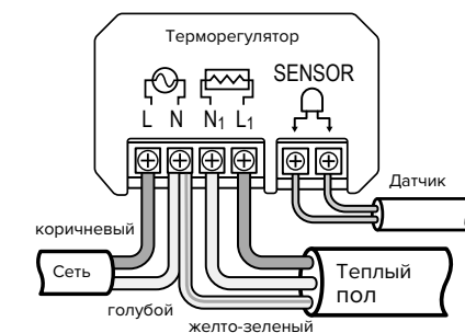
Подключение к 2-х проводной линии
