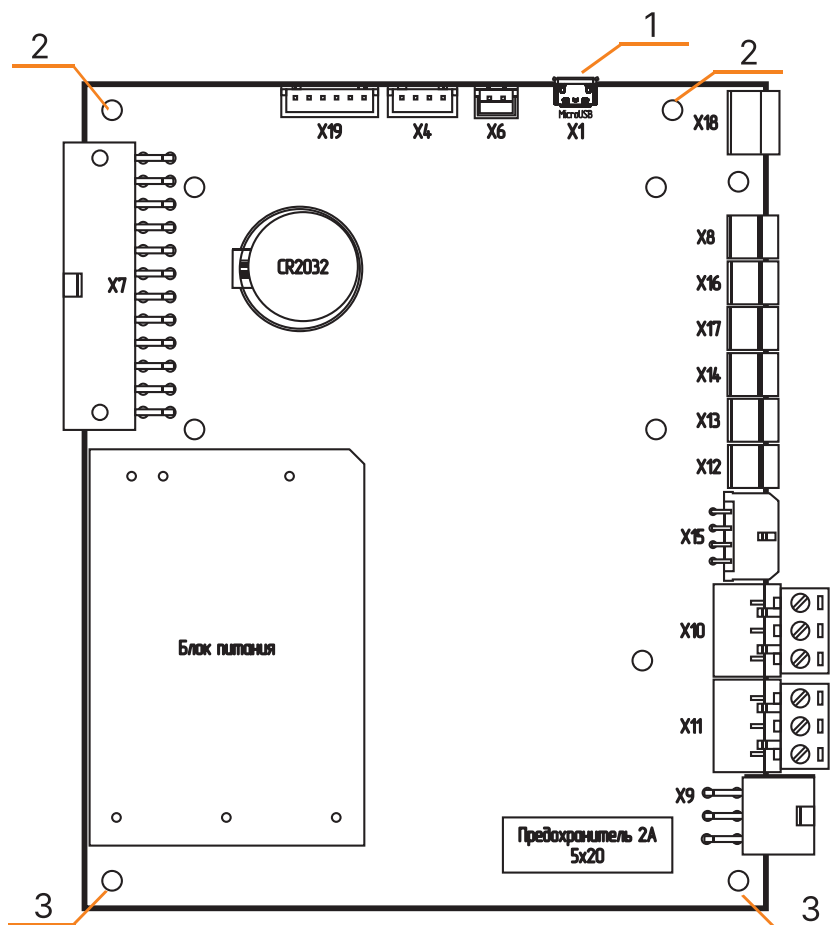
Рис.28 Плата контроллера
