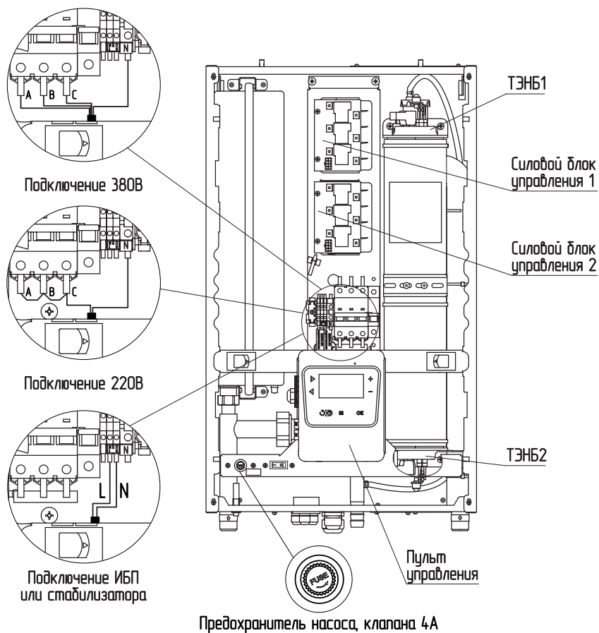
Рис.14 Органы управления электрического котла BAXI Ampera Plus 9-24 кВт
