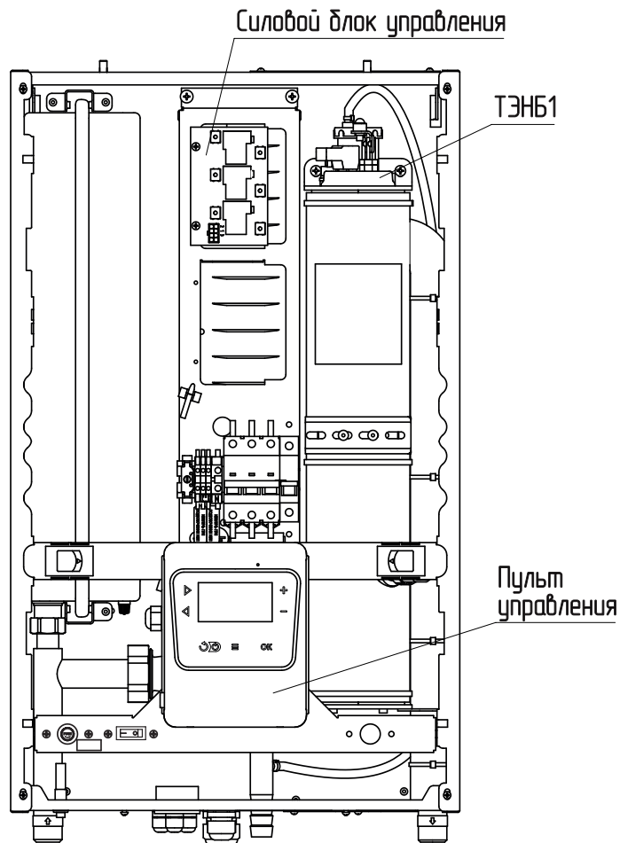
Рис.13 Органы управления электрического котла BAXI Ampera Plus 6 кВт
