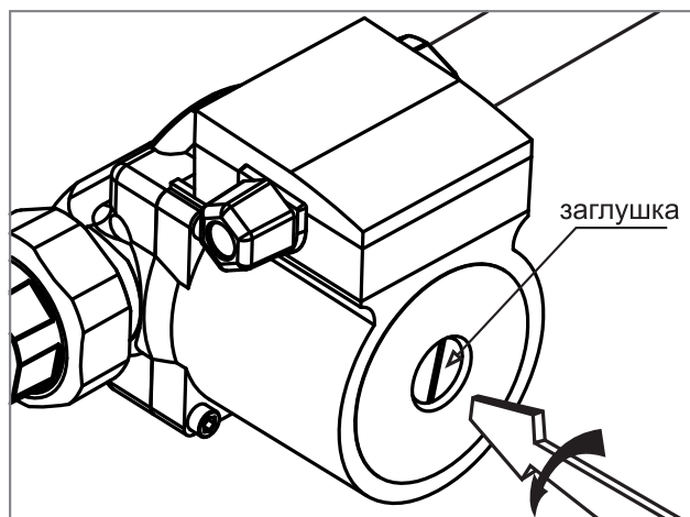
Рис.6 Удаление воздуха из насоса
