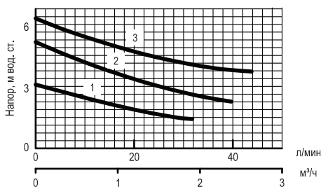
Диаграммы характеристик насосов АСР 25-60, АСР 32-60
