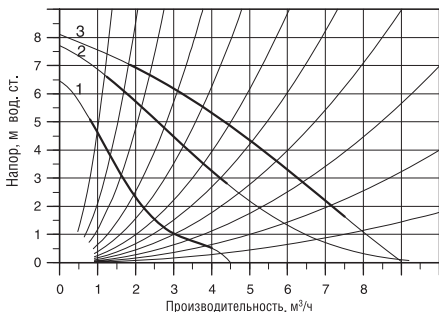
Диаграммы характеристик насоса АСР 25-80
