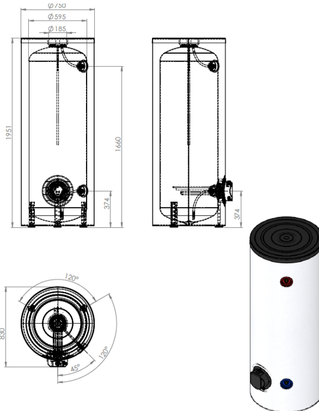
Afb. 1 – Afmetingen
