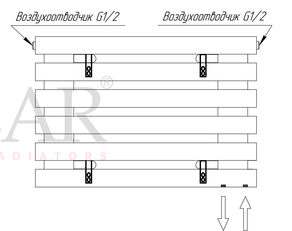
Подключение нижнее "биноклем" 150
