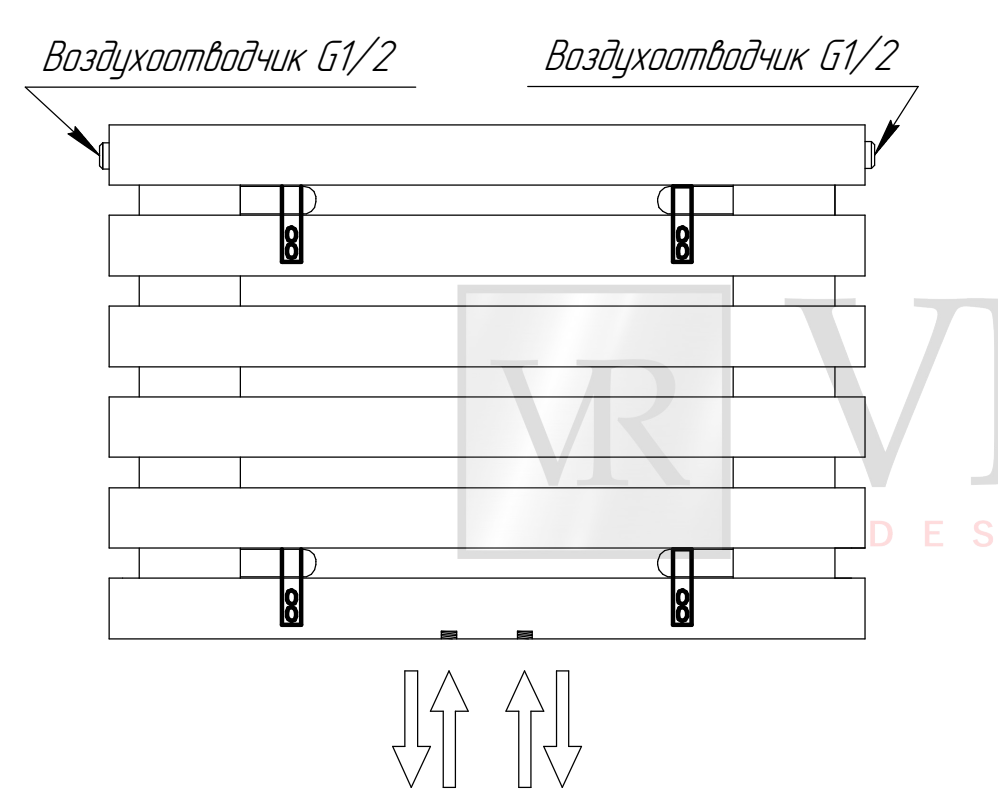
Подключение нижнее "биноклем" 050
