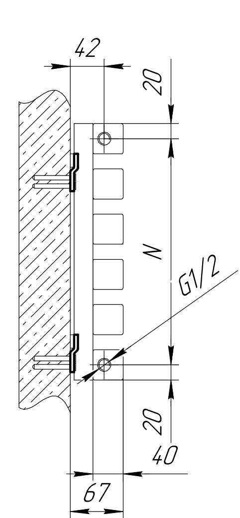
Подключение нижнее "биноклем" 150
