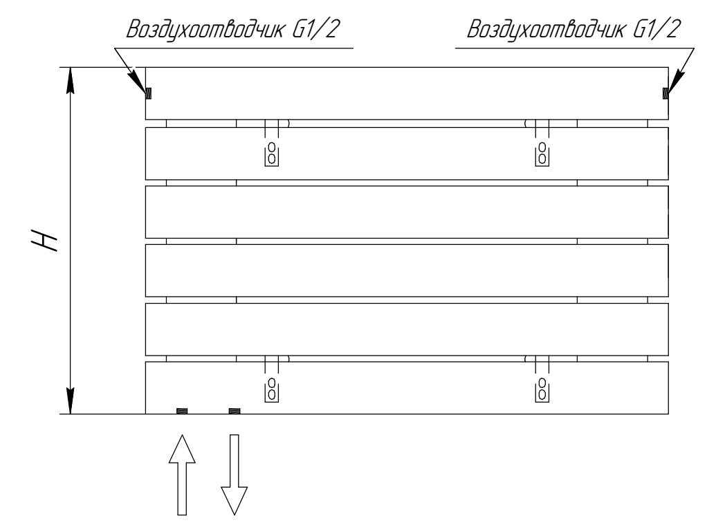
Подключение нижнее "биклем" 150
