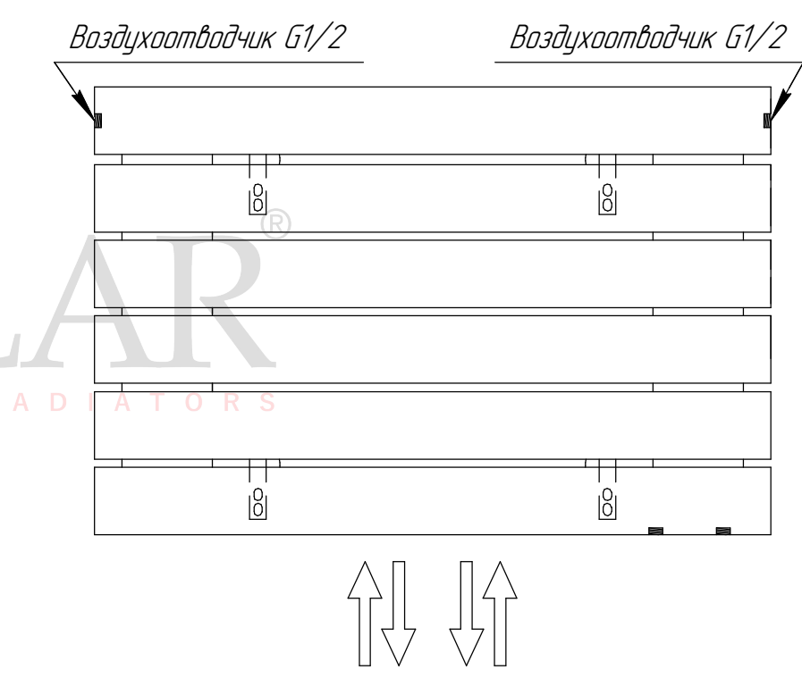
Подключение нижнее "биклем" 150
