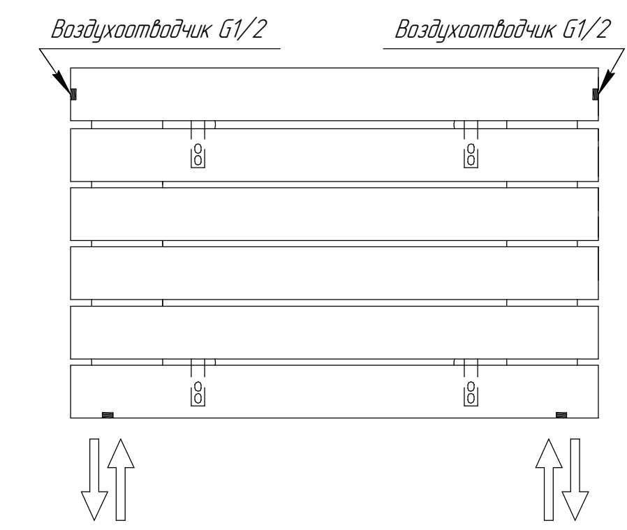
Подключение нижнее разнесенное 1П
