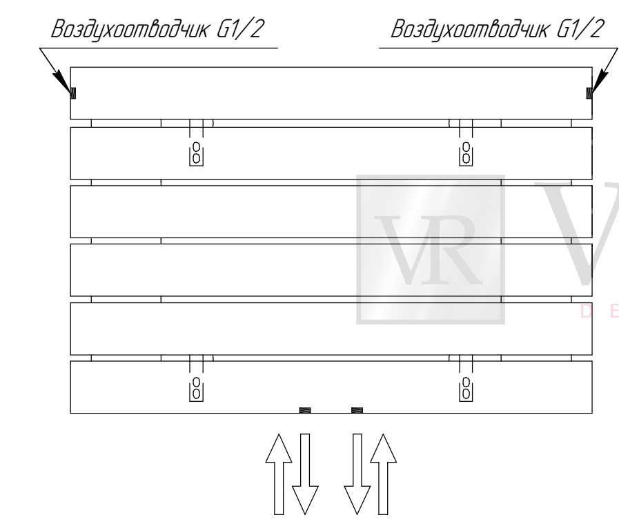
Подключение нижнее "биклем" 050
