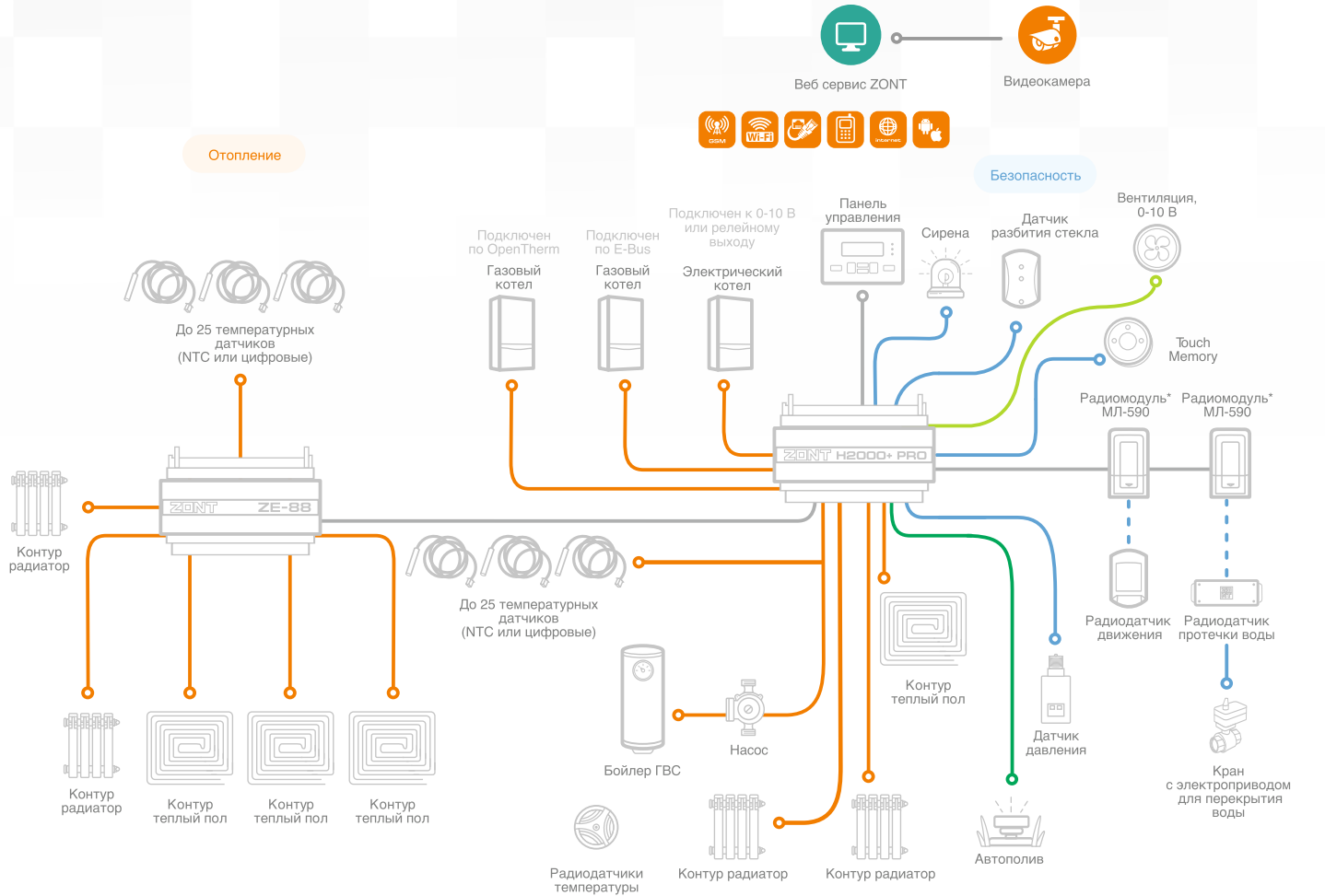
Пример инженерной системы на базе ZONT H2000+ PRO
