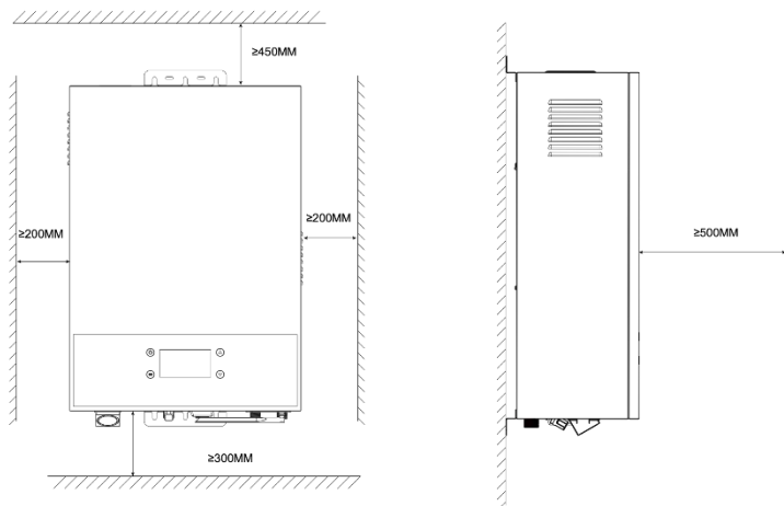
Рис. 5. Минимальные расстояния от электрического котла до поверхностей.
