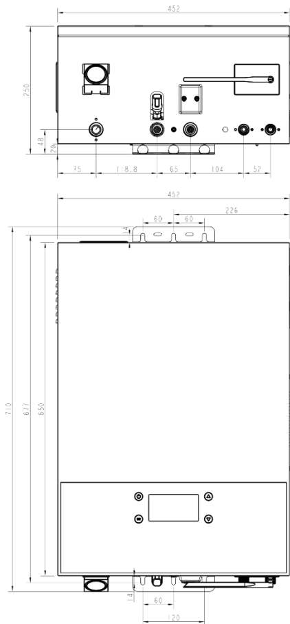
Рис.2. Габаритные размеры
