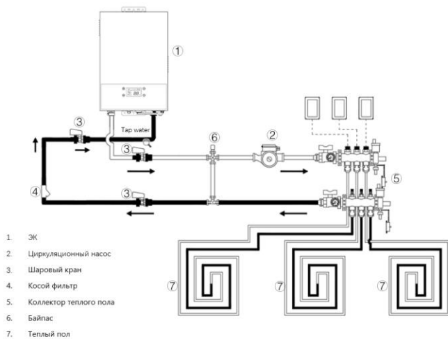
Рис. 8. Схема подключения «теплый пол + ЭК»
