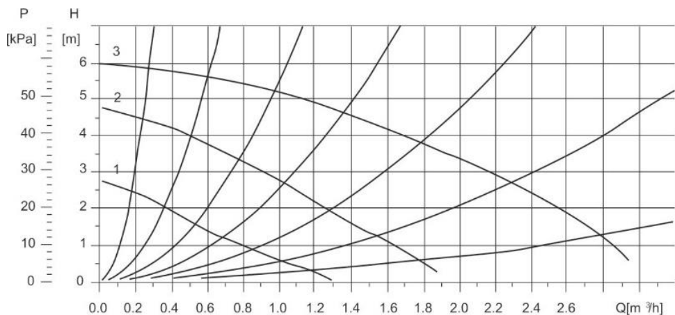
Рис. 15. Кривая характеристик давления насоса
