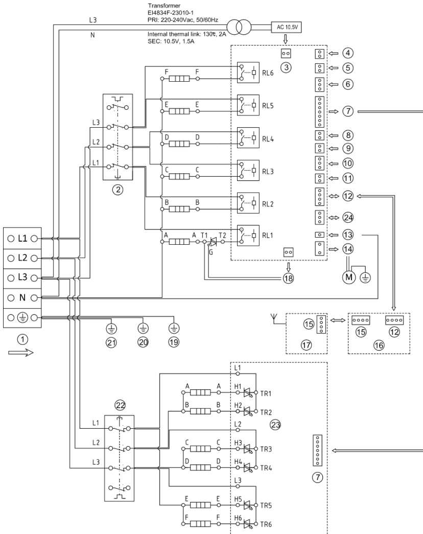
Рис.14. Электрическая схема
