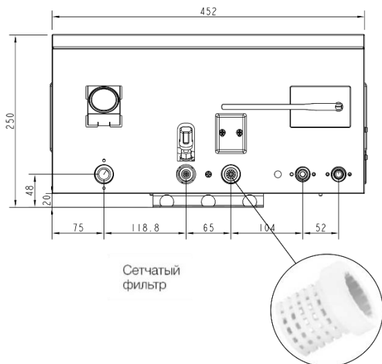
Рис. 16. Сетчатый фильтр
