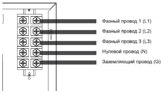
Рис.12. Подключение прибора
