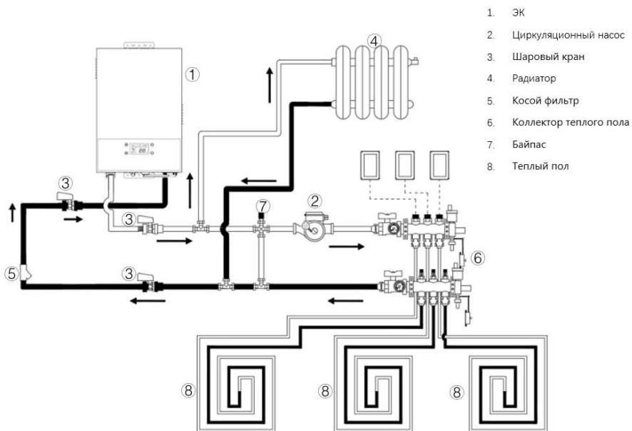
Рис. 9. Схема подключения «радиаторы + теплый пол + ЭК»
