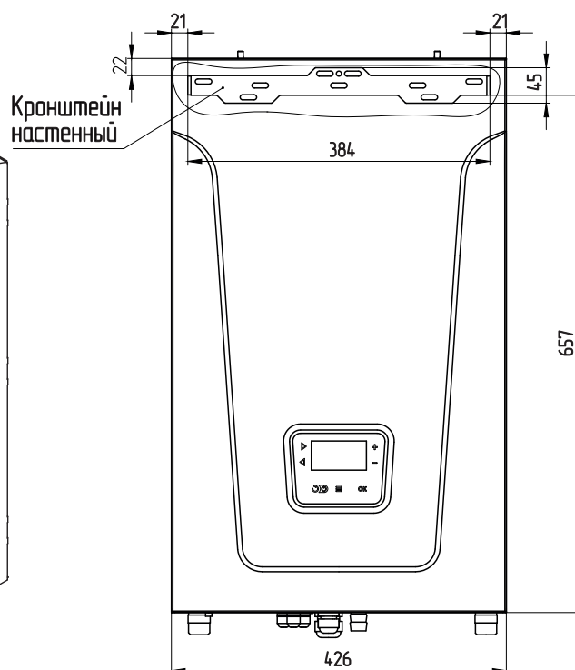
Рис.8 Positionирование котла относительно кронштейна
