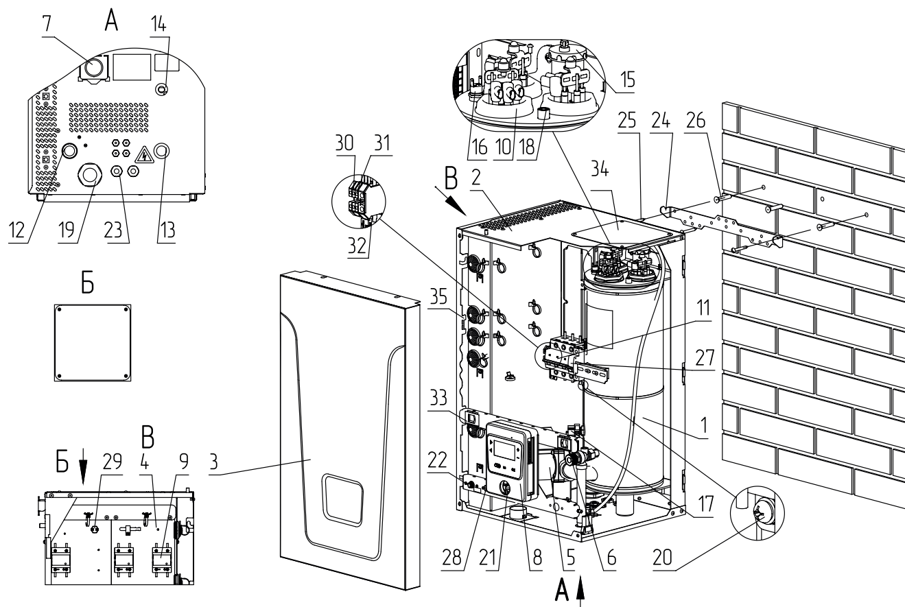
Рис.2 Конструкция котла
